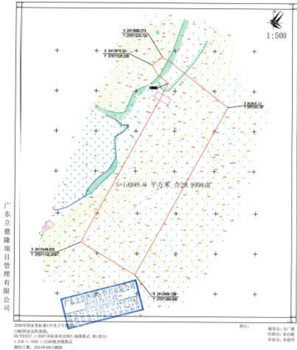
阳西县2024年度第三十三批次城镇建设用地勘测定界图 2413.383-37571.086
